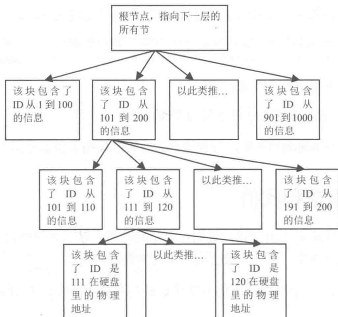
图 2.1 索引的结构图
