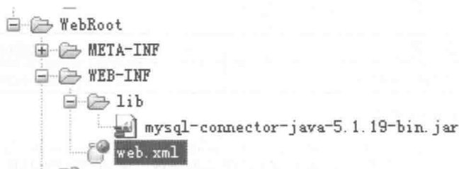
图 3.7 把 mysql-connector-java-5.1.19-bin.jar 放入 WEB-INF/lib 目录
