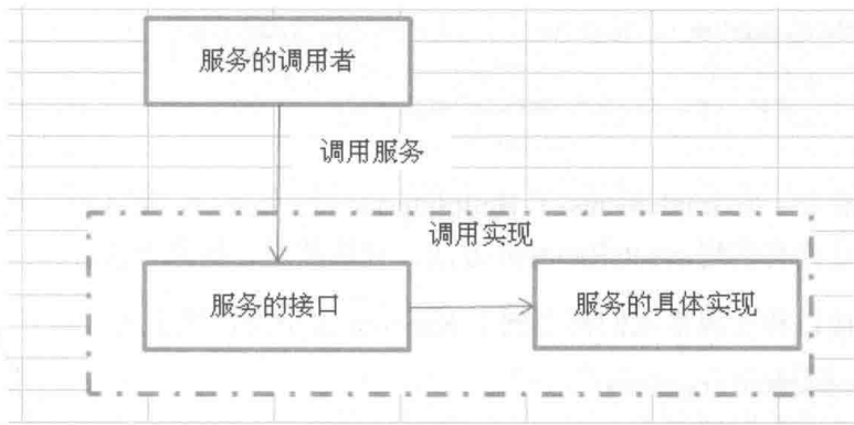
图 5.1 面向接口编程的调用方式
